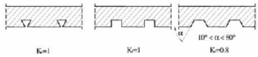
Figura 7.3 - Valori del coefficiente di forma delle lamiere grecate.
