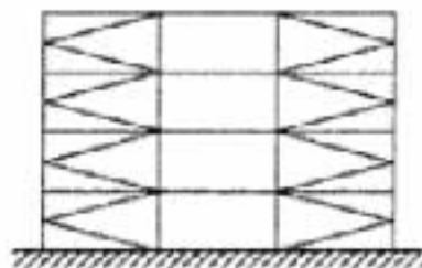
Controventi concentrici a K
