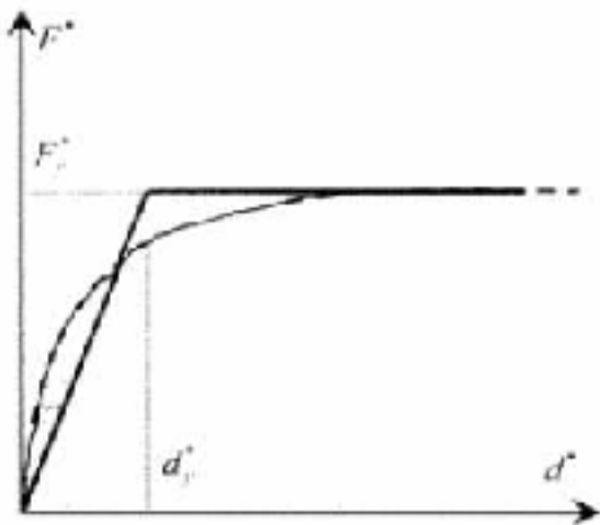
Figura 4.1 – Diagramma bilineare equivalente
