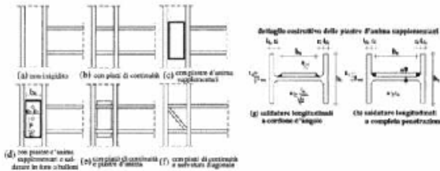
Figura 6.2. Dettagli costruttivi di pannelli nodali irrigiditi.
