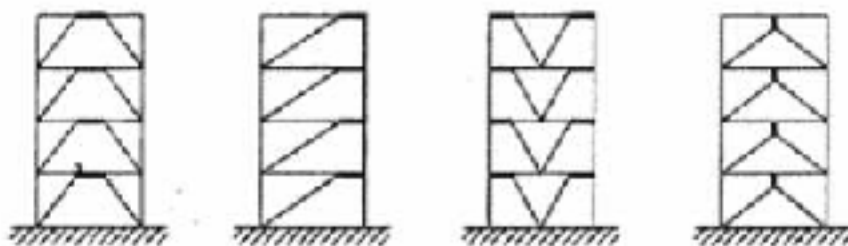
Controventi eccentrici
