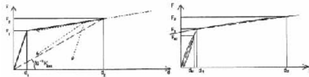
Figura 10.1 - Diagrammi forza - spostamento per dispositivi non lineari
