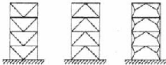
Controventi concentrici a V
