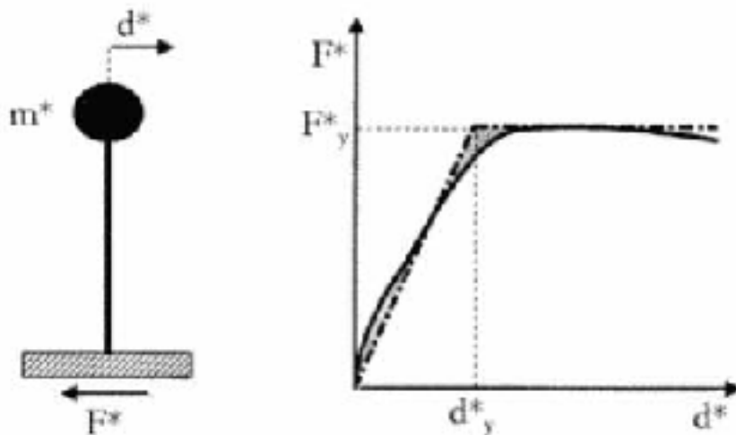
Figura 4.1 – Sistema e diagramma bilineare equivalente
