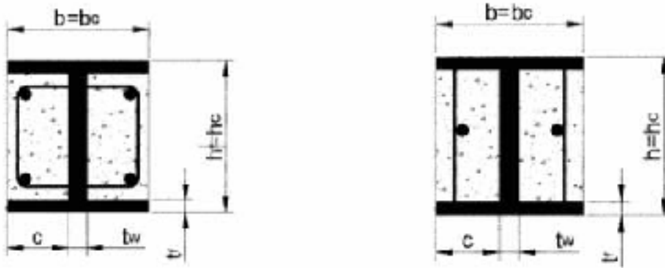
a) Staffe saldate all'anima
